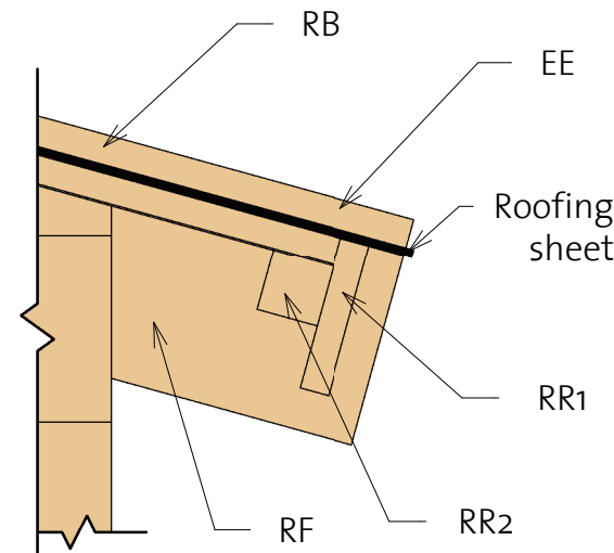
② Facia
